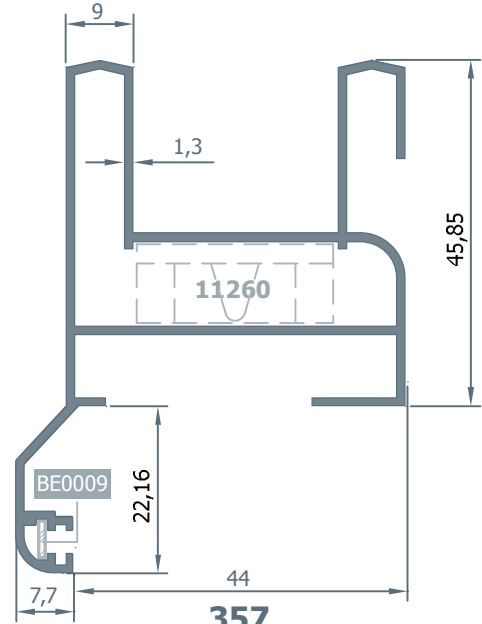
357 Kasa Profili 0.955 kg/m.
