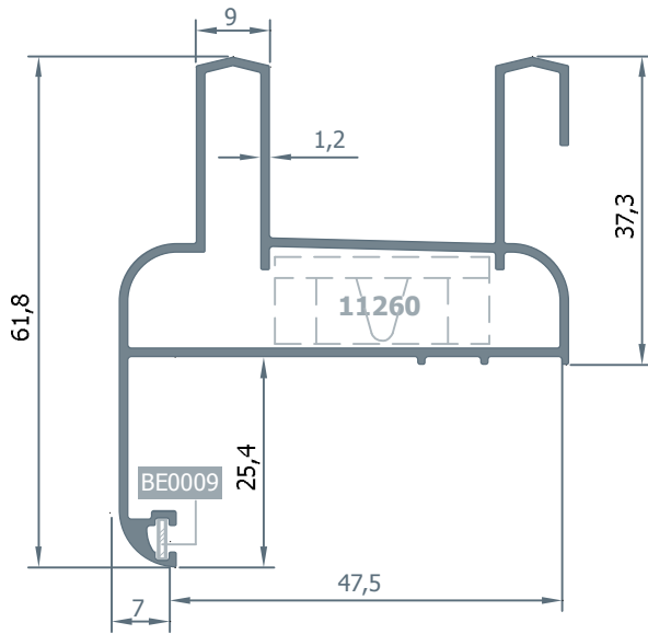
319.44 Kasa Profili 0.820 kg/m.
