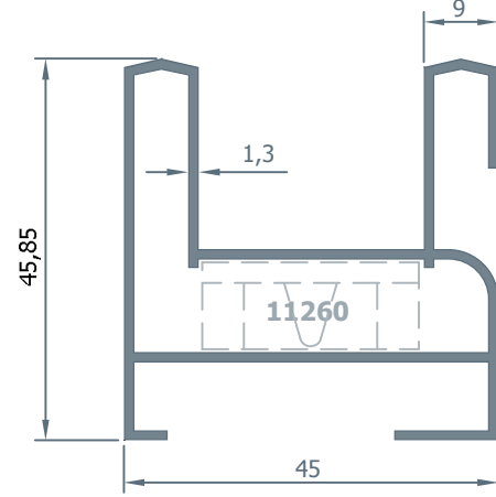
356 Kasa Profili 0.810 kg/m.
