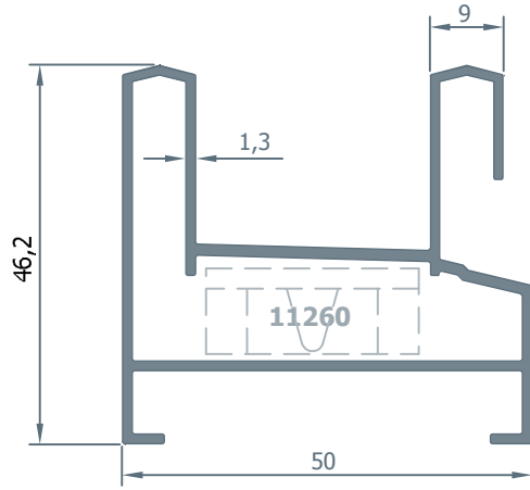
4410 Kasa Profili 0.850 kg/m.
